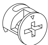
E x20 Ø15mm
